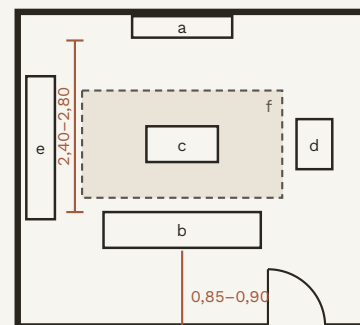
Schéma 02 · Implantation type, salon de 5,00 × 4,80 m, sans échelle. a cheminée · b canapé · c table basse · d fauteuil · e radassier · f tapis.
