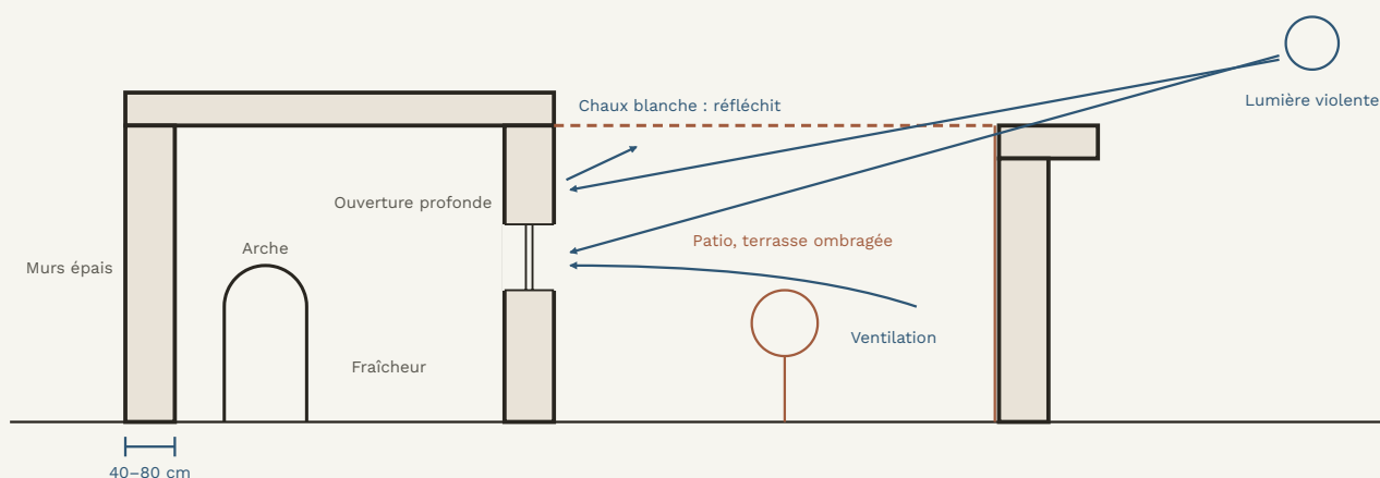
Schéma 01 · La maison du bassin, lecture climatique. Coupe de principe, sans échelle.
