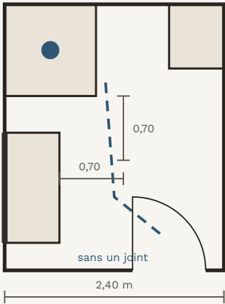
Salle de bain, 2,40 × 2,90 m, 7 m² SANS ÉCHELLE · DOUCHE À L'ITALIENNE, VASQUE DE PIERRE
