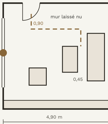
En plan
