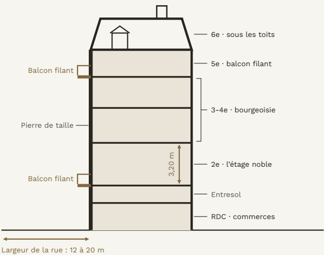
Schéma 01 · Coupe de principe de l'immeuble type, sans échelle.
