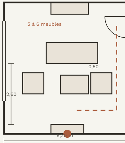
Séjour, 5,20 × 5,60 m, 29 m 2
