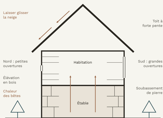
Schéma 01 · Le chalet, lecture climatique. Coupe de principe, sans échelle.
